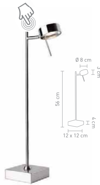
88424 tischleuchte metall chrom-matt table lamp metal chrome-matt
